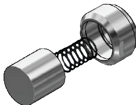
Conjunto botón accionamiento para válvula descarga CODIGO: R4303.3
